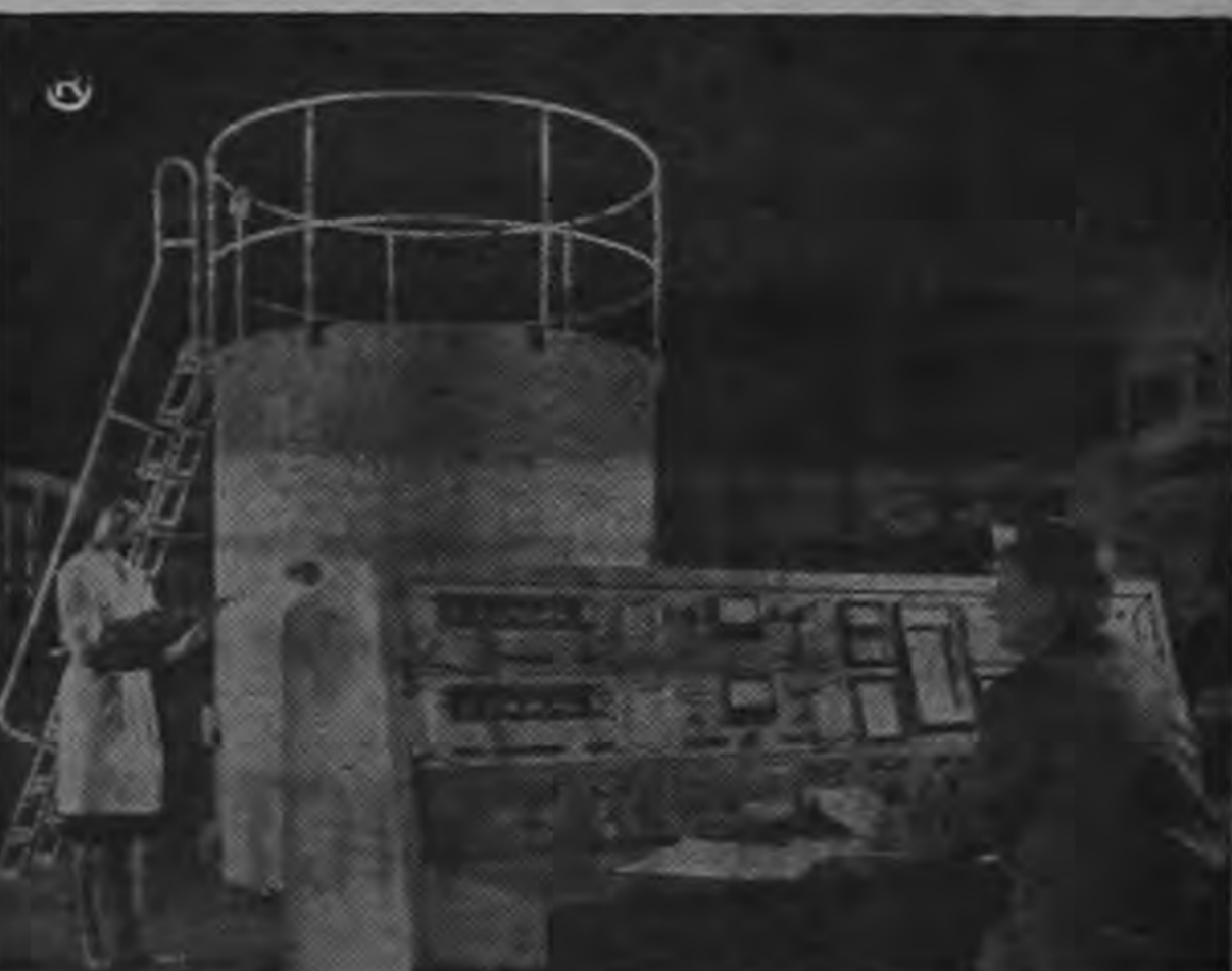
"También en el servicio de las centrales atómicas, la experiencia es la madre de la ciencia". Guiada por esta idea, Siemens-Schuckertwerke CONSTRUYE CONTINUAMENTE REACTORES NUCLEARES de pequeño tamaño, para la formación de científicos y técnicos. Los reactores creados para fines didácticos, pueden instalarse y prestar servicio, sin que ello origine grandes gastos ni suponga peligro alguno, en escuelas superiores o entidades de enseñanza técnica.
